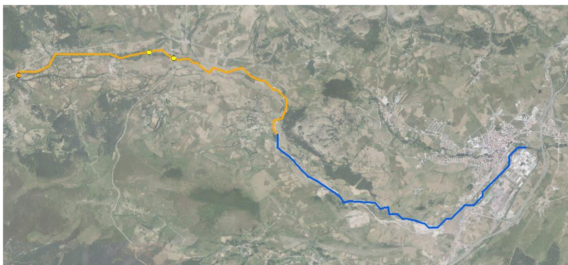
Figura 4. En azul se muestra el tramo de actuación del proyecto, correspondiente a las actuaciones continuas ejecutadas en los tramos medio y urbano (8 km). En color naranja se representa el tramo adicional en el que se mejora la continuidad, que discurre desde el obstáculo existente aguas arriba del último obstáculo permeabilizado en la obra y que se suma al tramo de actuación del río Híjar hasta su desembocadura en el Ebro para el cálculo de la longitud de río conectado. Los dos puntos amarillos indican la ubicación de los obstáculos permeabilizados con el proyecto.
